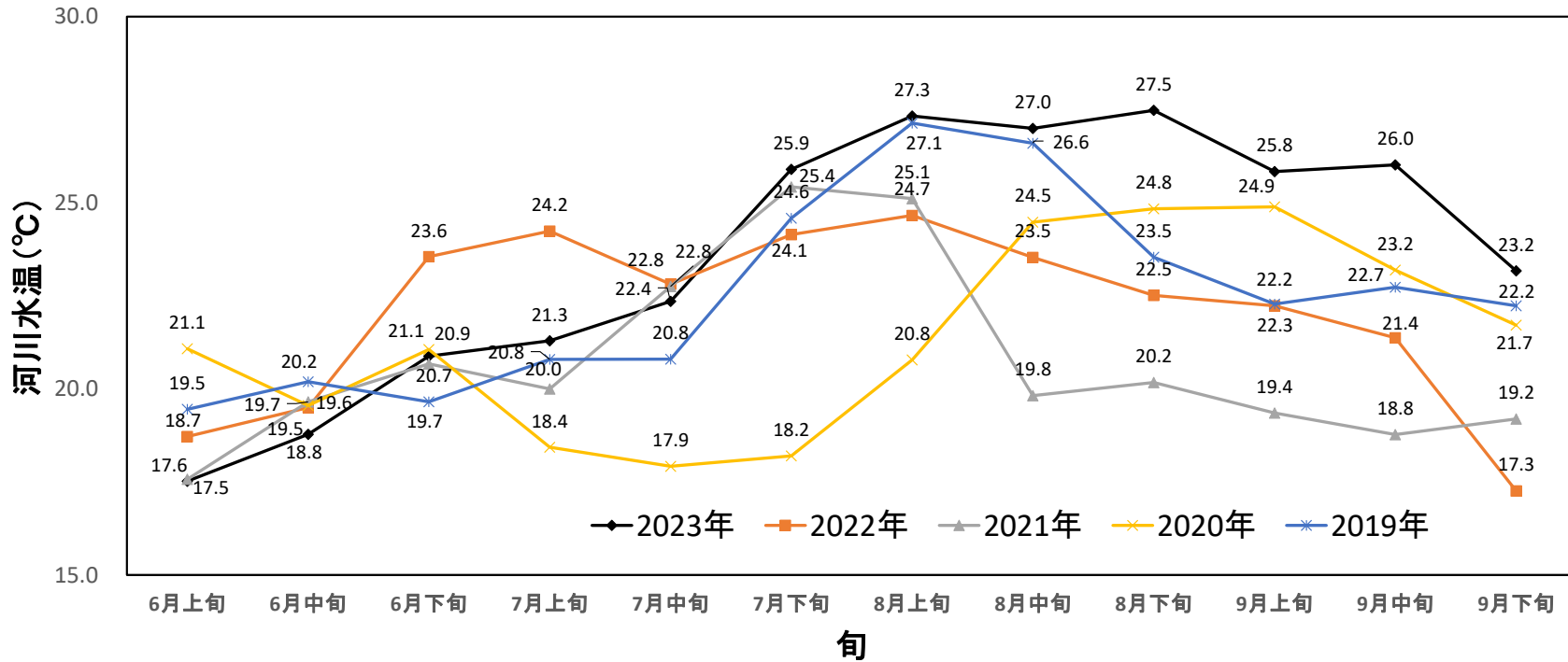
図.2023年～2019年 庄川本川河川水温 6月～9月旬毎平均水温比較
